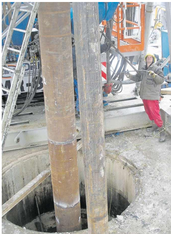
Bei der Firma Grob Gemüsebau in Schlattingen wurde erfolgreich nach Thermalwasser zum Beheizen von Gewächshäusern gebohrt. Bild: Caspar Hesse
